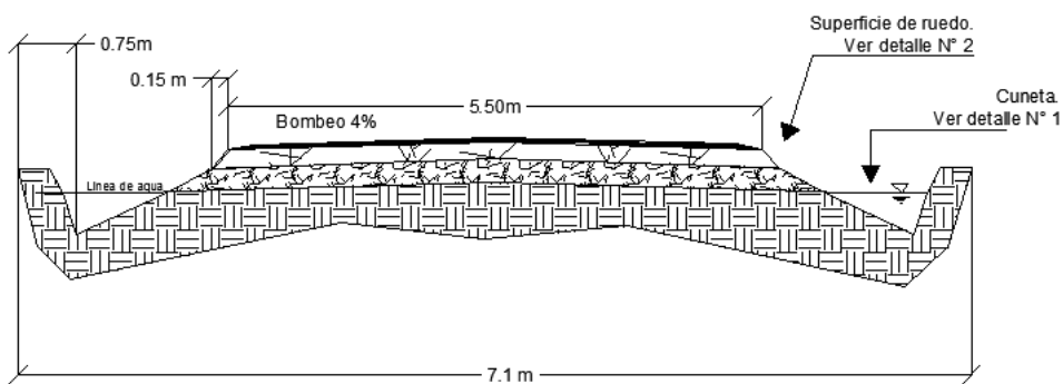
SECCIÓN TÍPICA 1 Esc: 1:75
