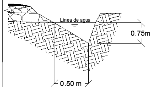
Detalle N° 1. Sección de cuneta Esc: 1:50
