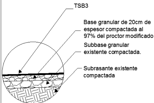
Detalle N° 2. Superficie de ruedo Esc: 1:50
